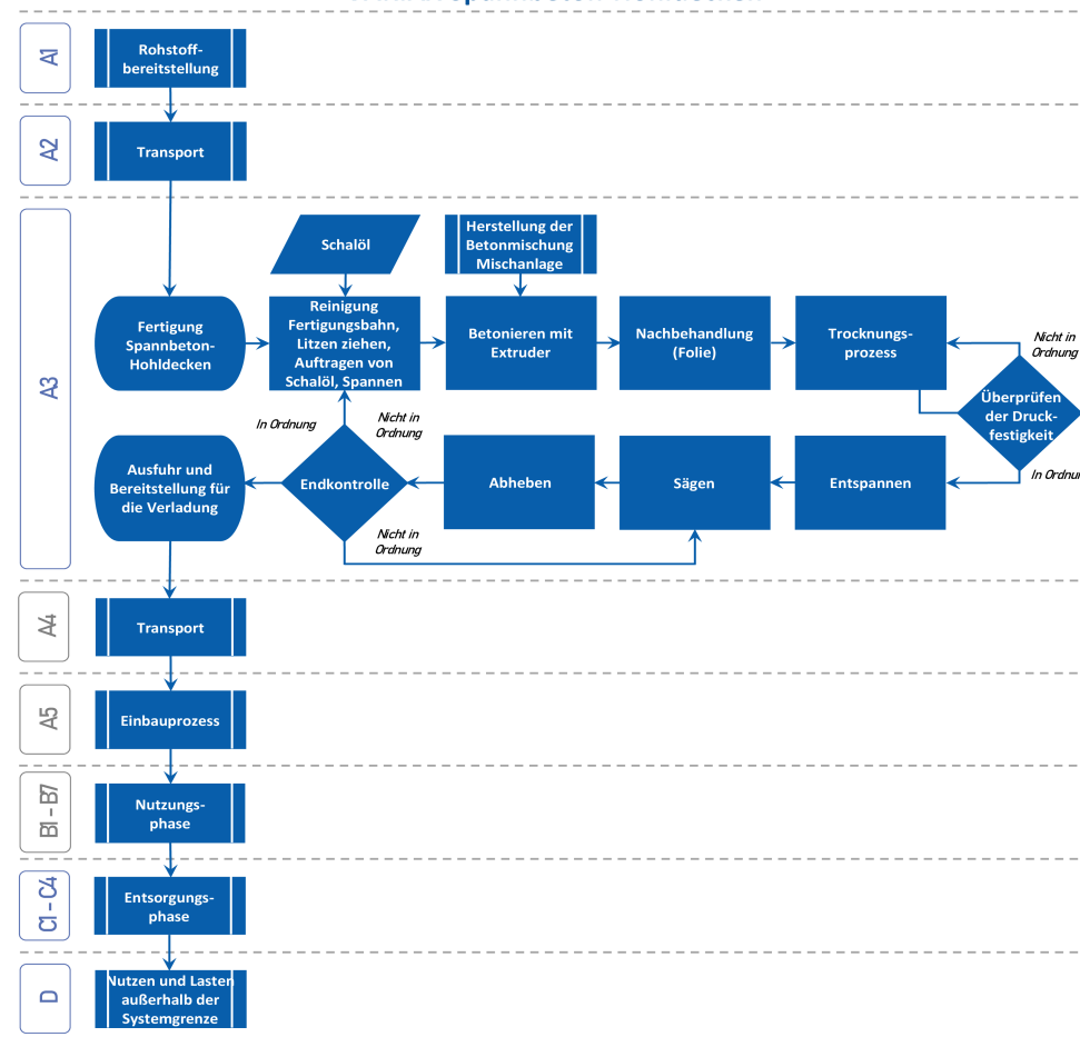
Produktflussdiagramm VARIAX Spannbeton-Hohldecken
